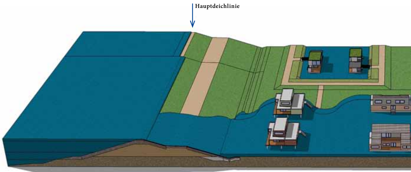
Einsatz von adaptiven Bauweisen wie Schwimmenden Häusern, Amphibischen Häusern und Pfahlhäusern
