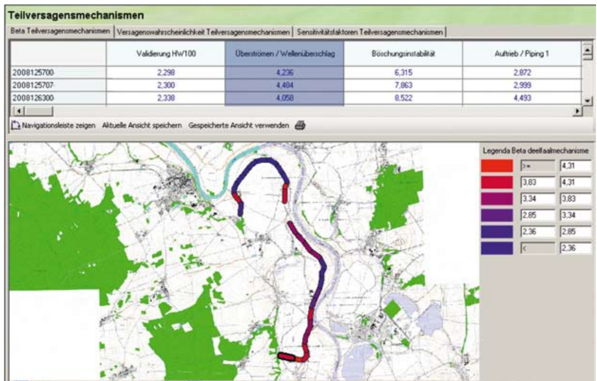
→ ABB. 31 Benutzeroberfläche des Programms PC-Ring für eine Deichstrecke an der Elbe
