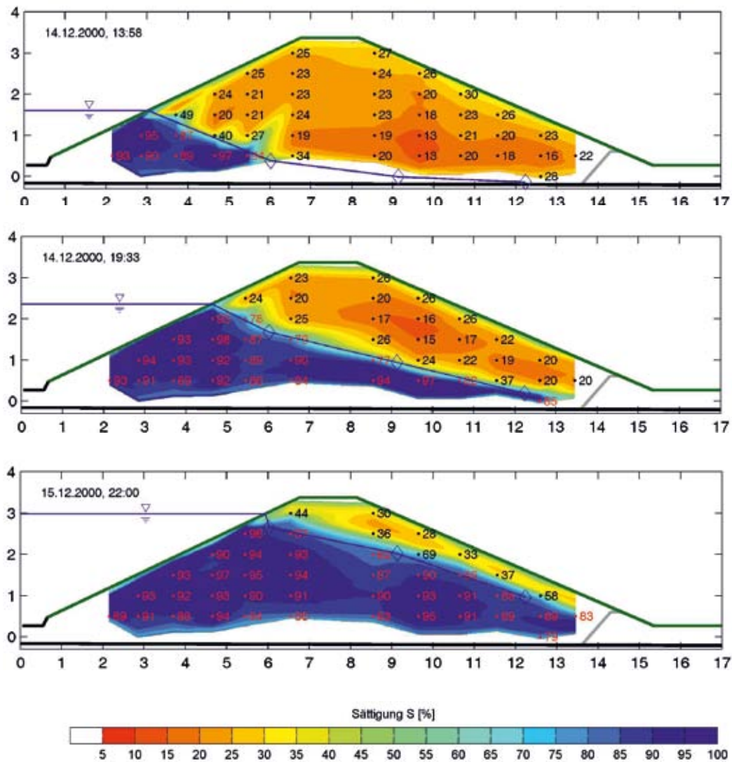
→ ABB. 29 Mit Flachbandkabeln gemessene Feuchteverteilung innerhalb eines Deichkörpers als Sättigungsverteilung während eines Einstauversuches
