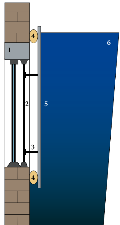
→ ABB. 33 Prinzipskizze des Schottsystems mit selbst dichtender Wassersperre
