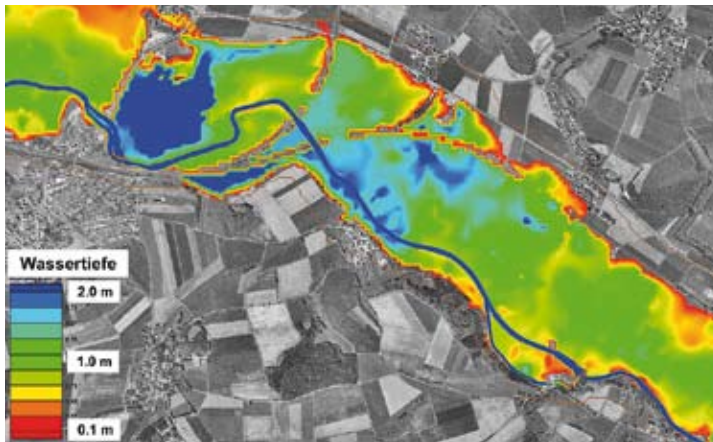
→ ABB. 7 Einzugsgebiet des Oberen Mains bis zum Pegel Kemmern mit Überschwemmungsflächen
