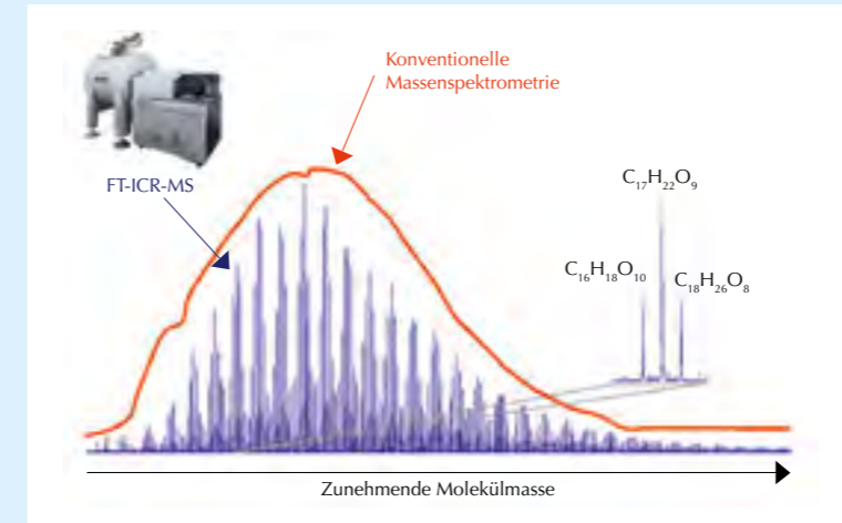
Fourier Transformation Ionen Zyklotron Resonanz Massenspektrometrie (FT-ICR-MS): Im Gegensatz zu konventionellen massenspektrometrischen Methoden (rotes Spektrum) können in jeder einzelnen Probe tausende Substanzen detektiert, getrennt und die zugehörigen Elementzusammensetzungen (Summenformeln) ermittelt werden. Grafik: B. Koch, AWI
